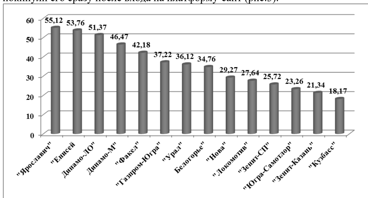
Рис.4. Показатель отказов (%)
